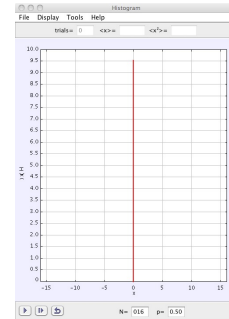
Stp_RandomWalk 1D.jar
