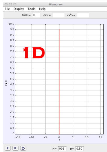
Stp_RandomWalk1D.jar
