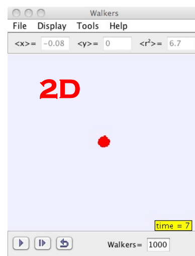
Stp_RandomWalk2D.jar
